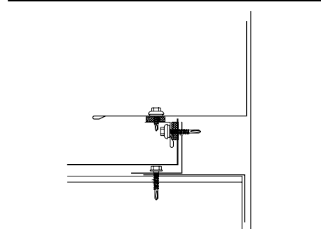
Rakewall Off Module Option
