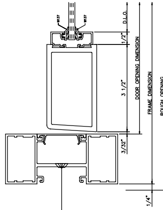
300 LEFT DOOR STILE
