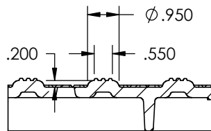
SECTION D-D SCALE 1 : 4
