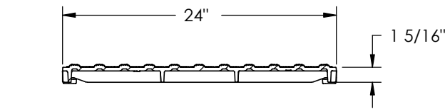
SECTION A-A
