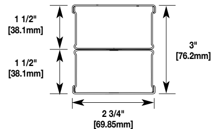
30TP-4V / 30TC-4V**
