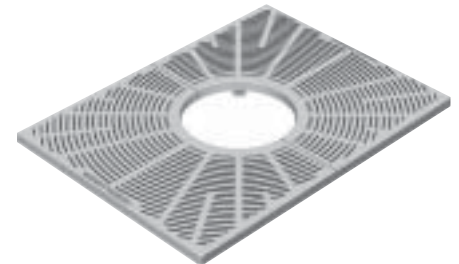
R-8814-A • 36" x 48"
