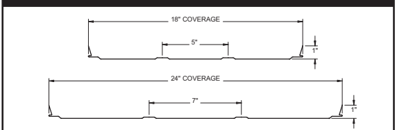
Grand Batten
