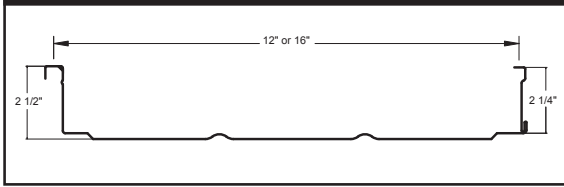
Stand 'N Seam®
