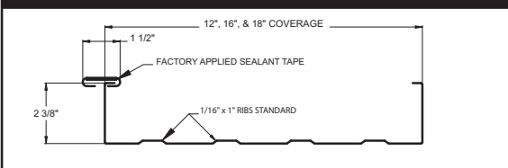
T-Rib
