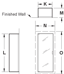
TRIMLESS
