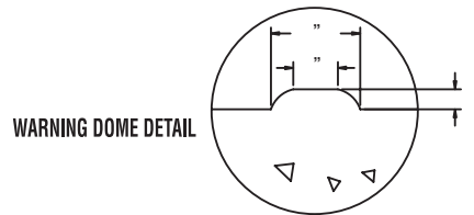
12" NOMINAL ADA PAVER
