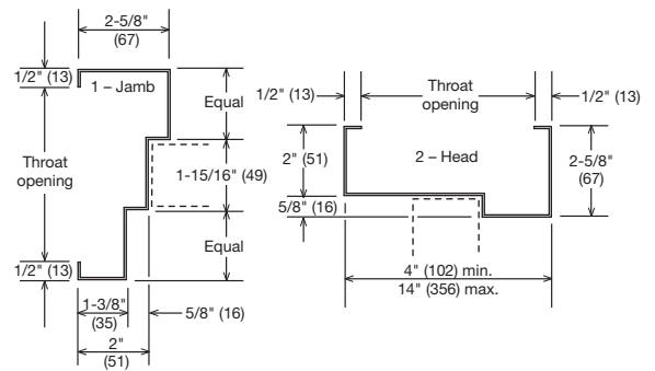
Section 1 Jamb
